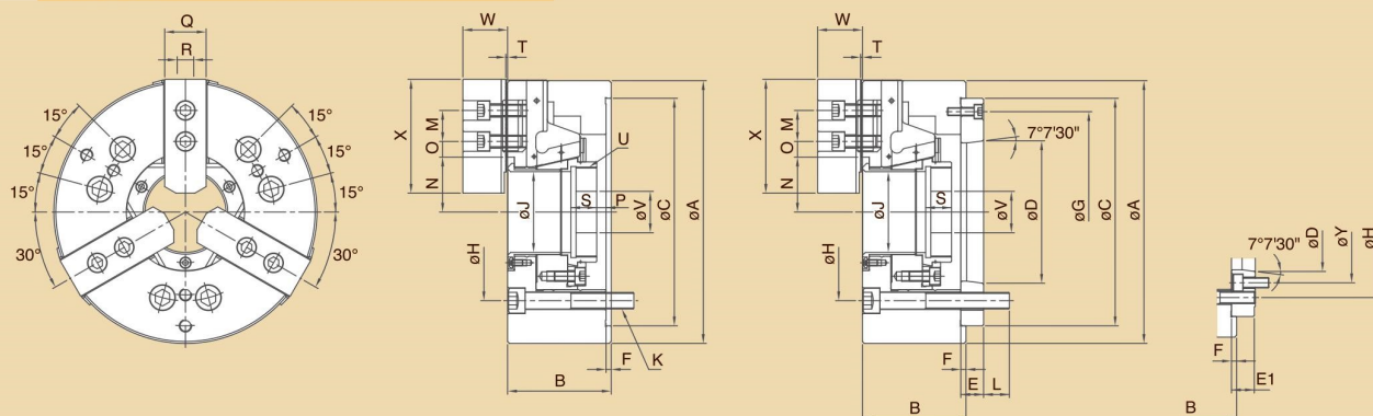
尺寸圖 » Dimensions
